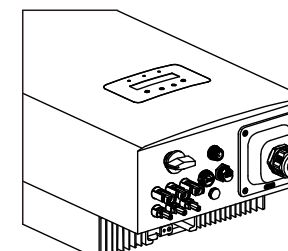
▲ Figura 4.17 Desmontar a tampa de terminal CA
