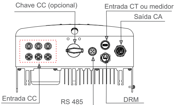
Figura 1.2 Vista lateral inferior
