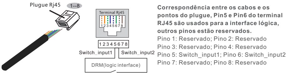
Figura 4.29 Retire a camada de isolamento e conecte ao plugue Rj45
