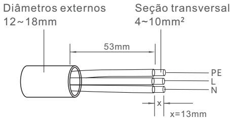
Figura 4.13 Fios CA descascados
