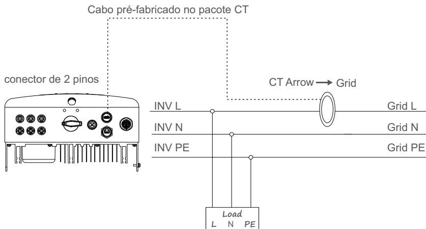
Figura 4.27 Sensor inteligente
