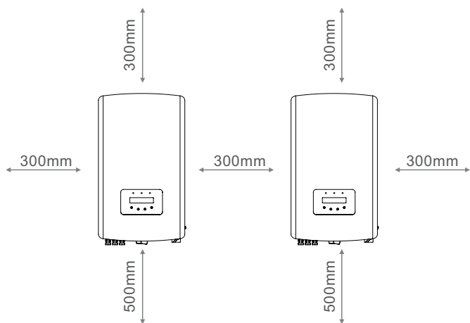
Figura 4.2 Folga de montagem do inversor
