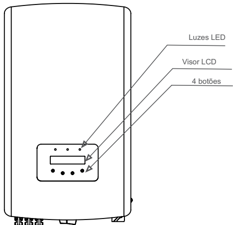
Figura 1.1 Vista lateral frontal
