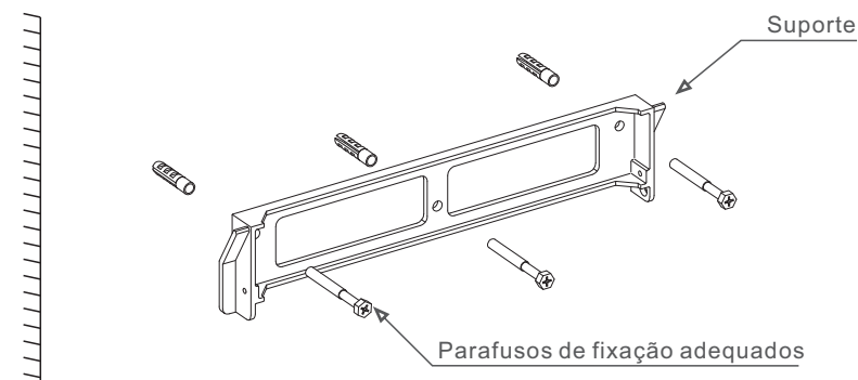
Figura 4.4. Montagem na parede do inversor
